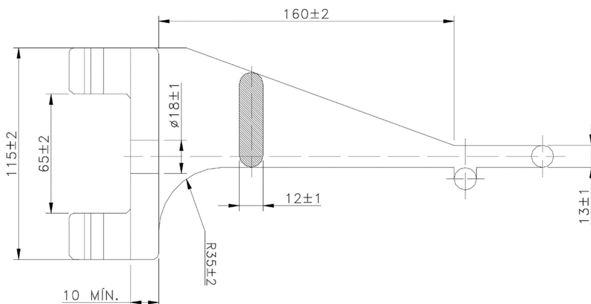
Figura 2 – Cruzeta Universal para Poste Circular – Vista Lateral
