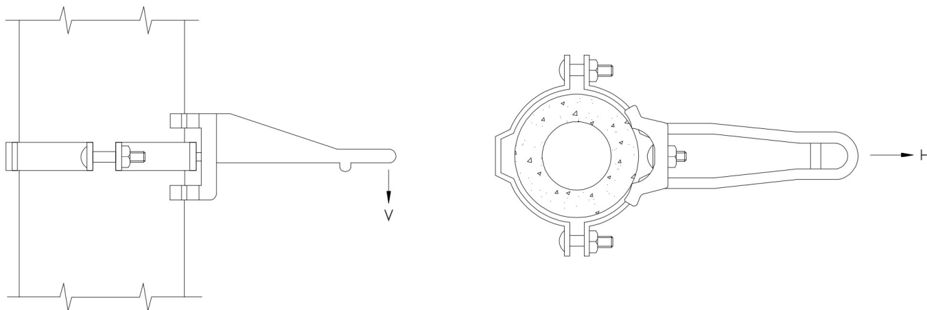
Figura 3 - Detalhe 1 - Indicação de esforços aplicados ara execução do ensaio em Poste Circular
